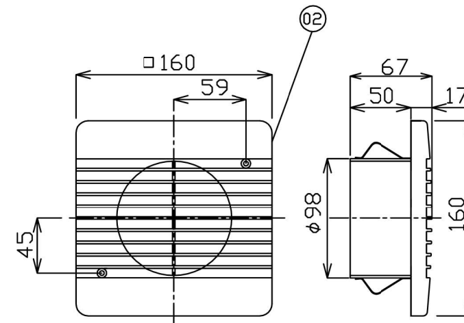
副吸込口パネル
