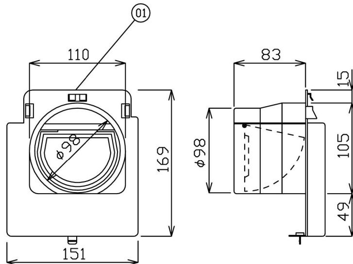
ダクト接続口（副吸込口側）
